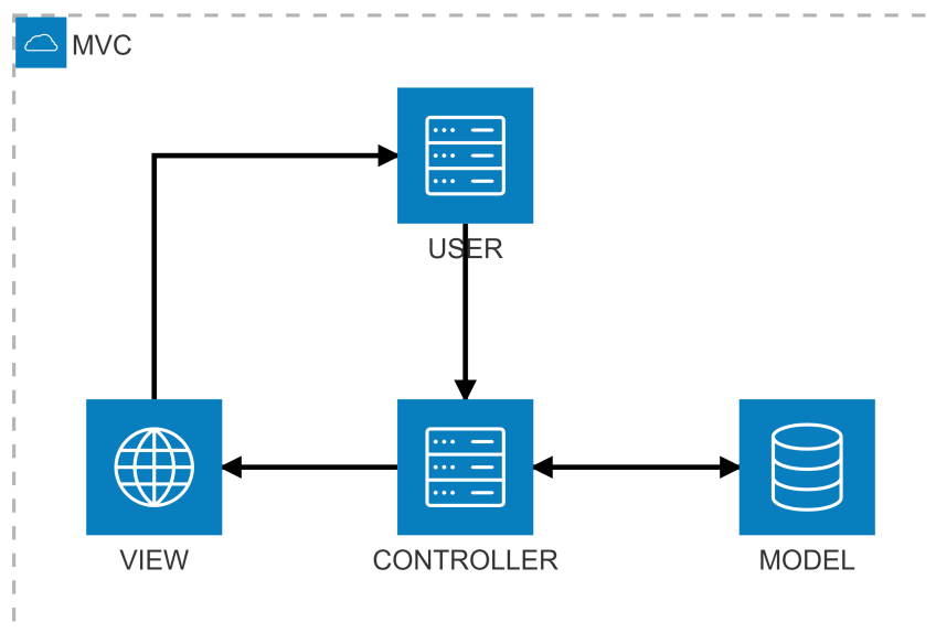
Figura 1 – Arquitetura MVC
