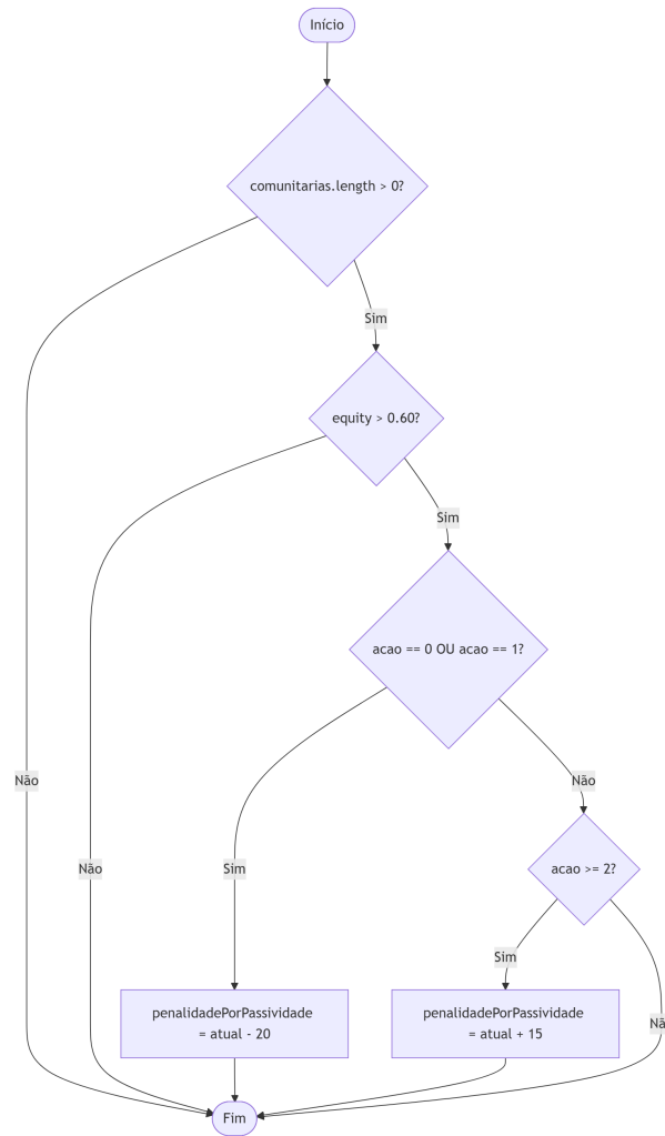
Figura 2 – Fluxograma do sistema de penalidade por passividade
